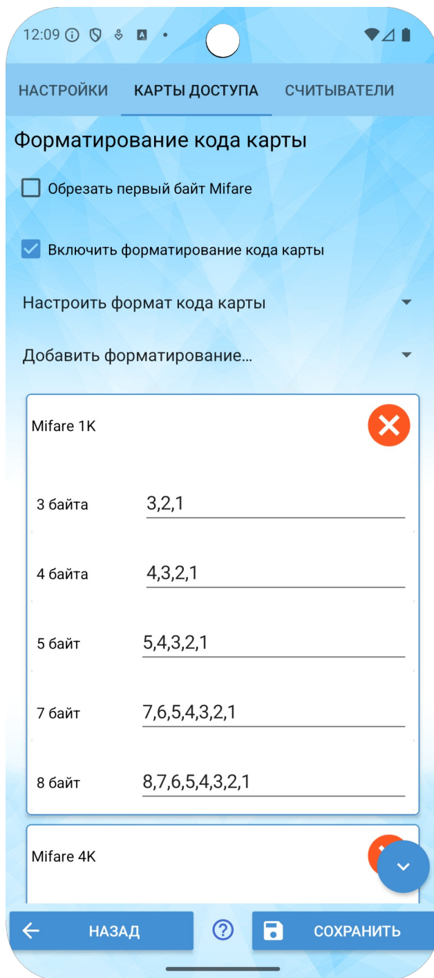
Рис. 20: Настройки форматирования кода карты
