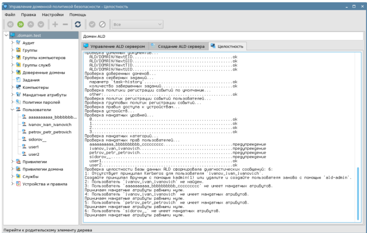
Рис. 10. Сведения о целостности домена ALD
