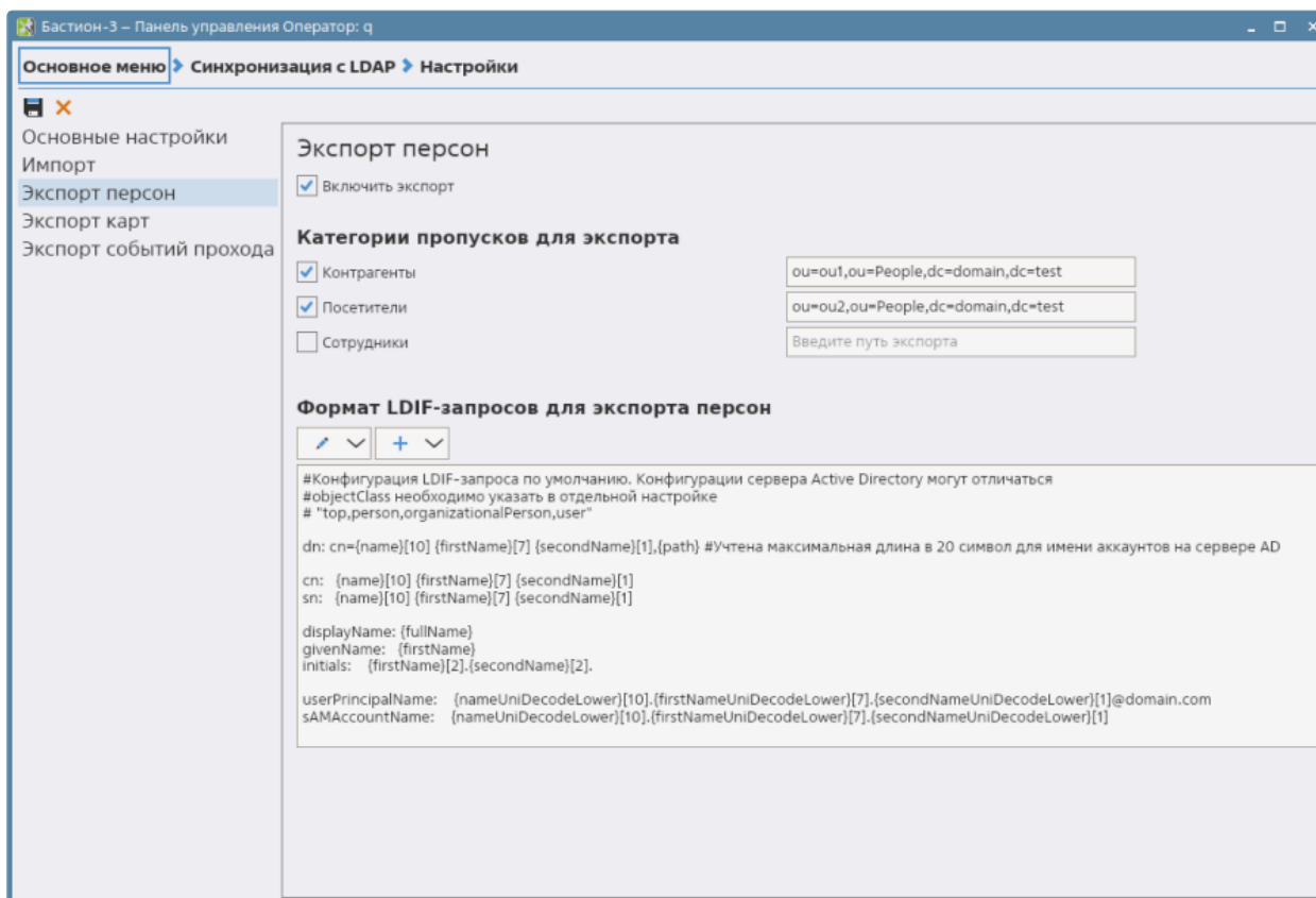
Рис. 5. Окно «Экспорт персон»
