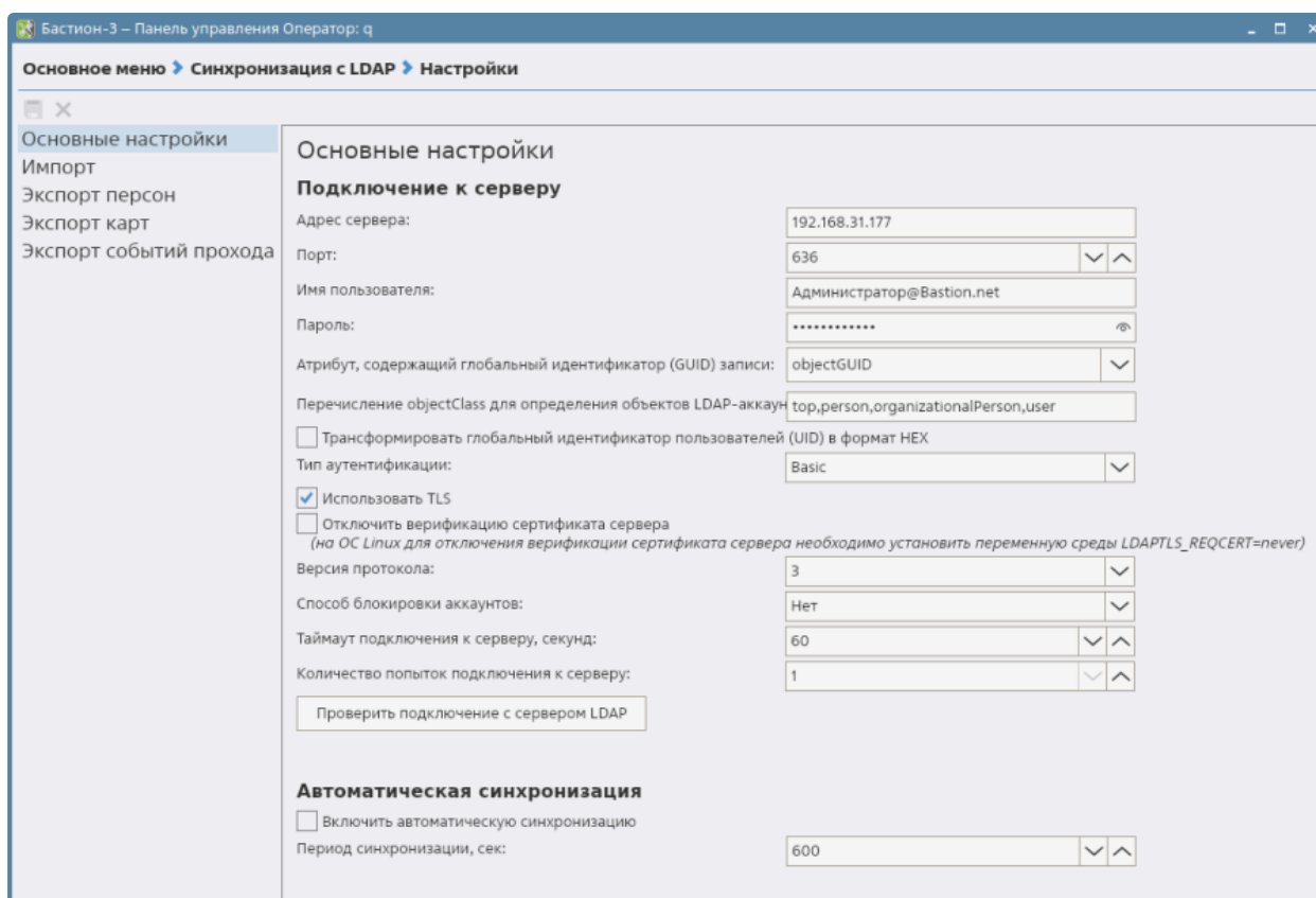
Рис. 3. Окно «Основные настройки»
