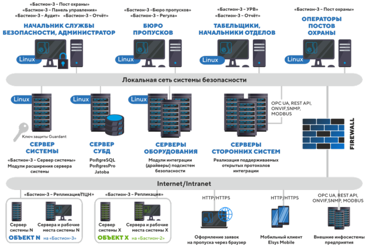
Рис. 1. Структура сети ПК «Бастион-3»
