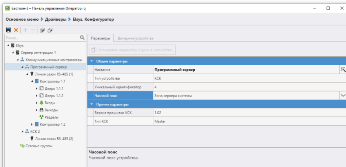
Рис. 1. Главное окно конфигуратора драйверов
