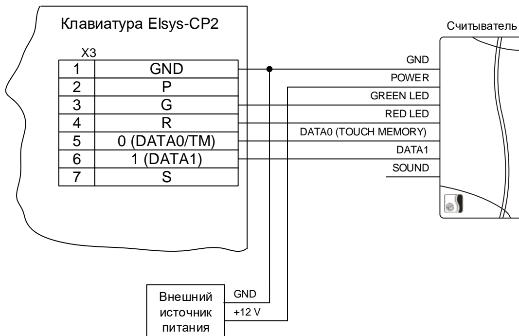
Рисунок 5. Подключение считывателя с питанием от клавиатуры
